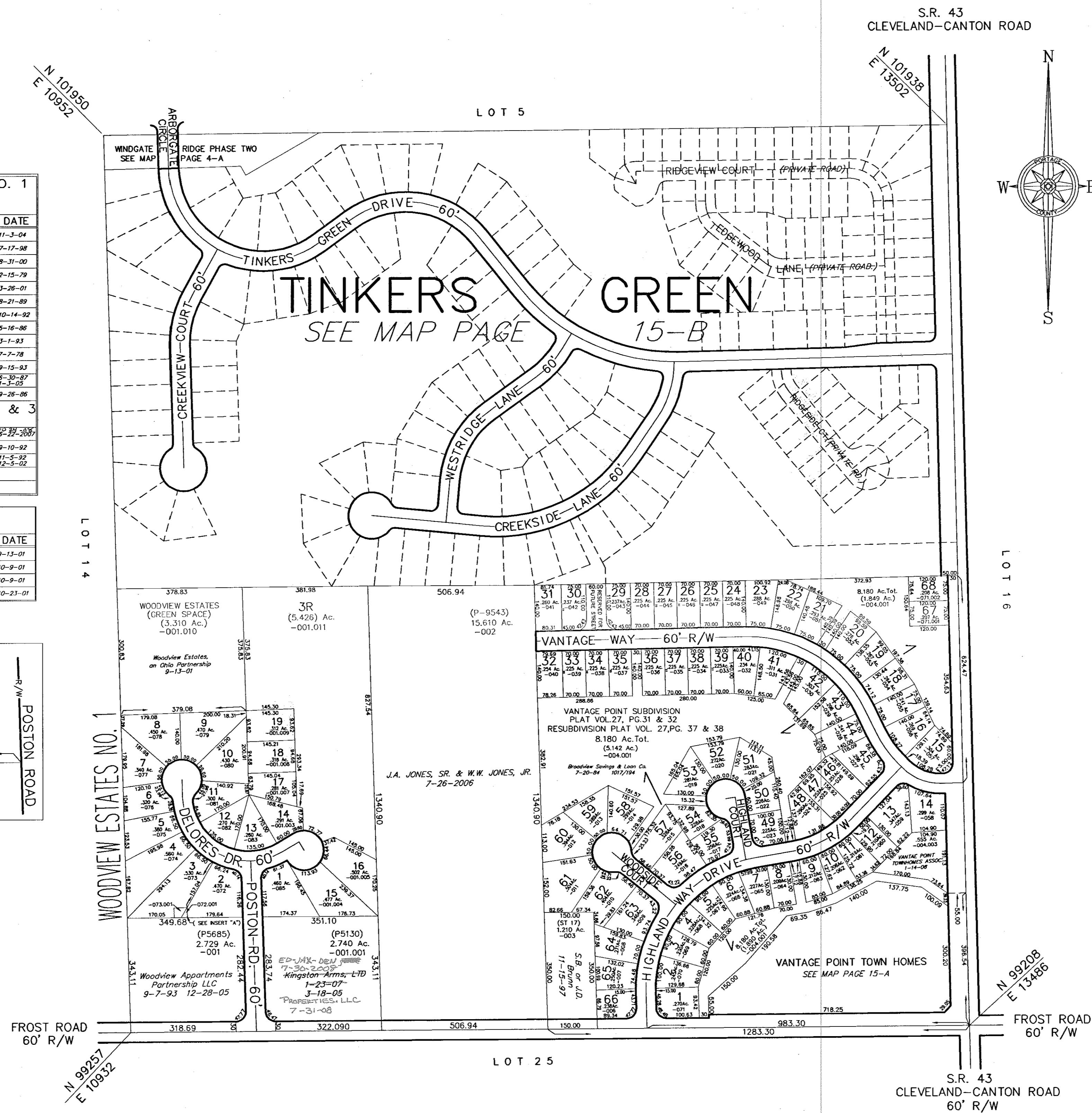
VANTAGE POINT SUBDIVISION PLAT VOL.27, PG.31 & 32 RESUBDIVISION PLAT VOL. 27, PG. 37 & 38
